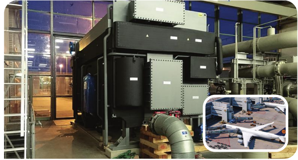
독일 Munich International Airport 저온수2단 흡수냉동기 975usRT
