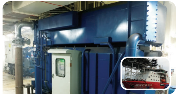
중국 Novenco Marine&Offshore 선박용 저온수 흡수냉동기 156usRT
